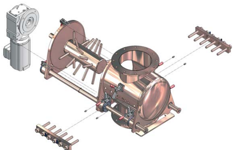
Enkele pennenbreker welke snelreinigbaar is uitgevoerd. Goed inzetbaar bij bedrijven waar veel productwissels aan de orde zijn.
